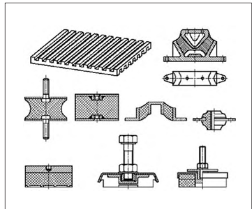
Figura 13.4: Alcuni esempi di diverse conformazioni di molle elastomeriche.
