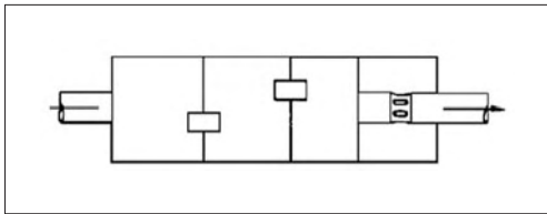
Figura 23.2: Silenziatore a riflessione e risuonatore.
