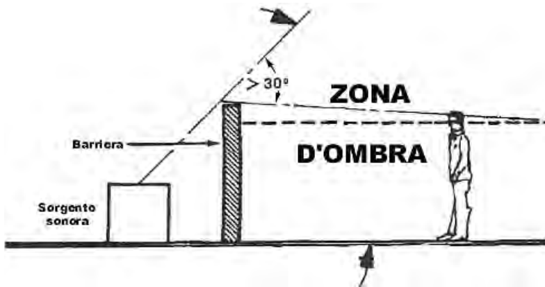
Figura 6.7: Come criterio generale, l'effetto d'attenuazione di una barriera sarà tanto maggiore, quanto maggiore di 30° sarà l'angolo relativo al punto d'ascolto situato nella zona d'ombra.
